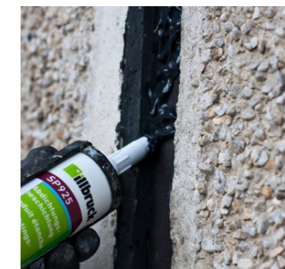
Aplikace tekuté hydroizolační membrány na komprimační pásku
