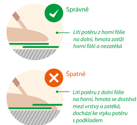
2 Lití podlahy
